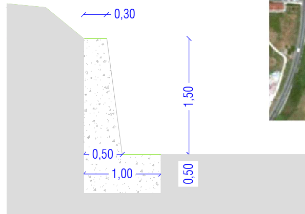
scala 1:50
